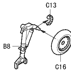
<<右侧主起落架>> Right main undercarriage
