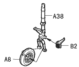
<<前起落架>> Nose undercarriage
