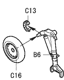
<<左侧主起落架>> Left main undercarriage
