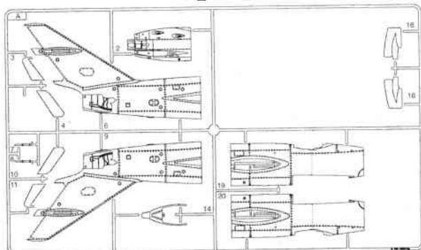
部件图 (Parts)
