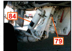
Train droit - vue avant Right landing gear - front view
