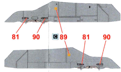
4x Pylônes sous voilure (points internes) 4x underwing pylons (inner stations)
