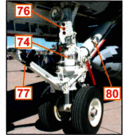
Train avant - vue avant Front landing gear - front view
