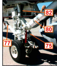
Train avant - vue arrière Front landing gear - rear view
