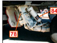
Train gauche - vue avant Left landing gear - front view
