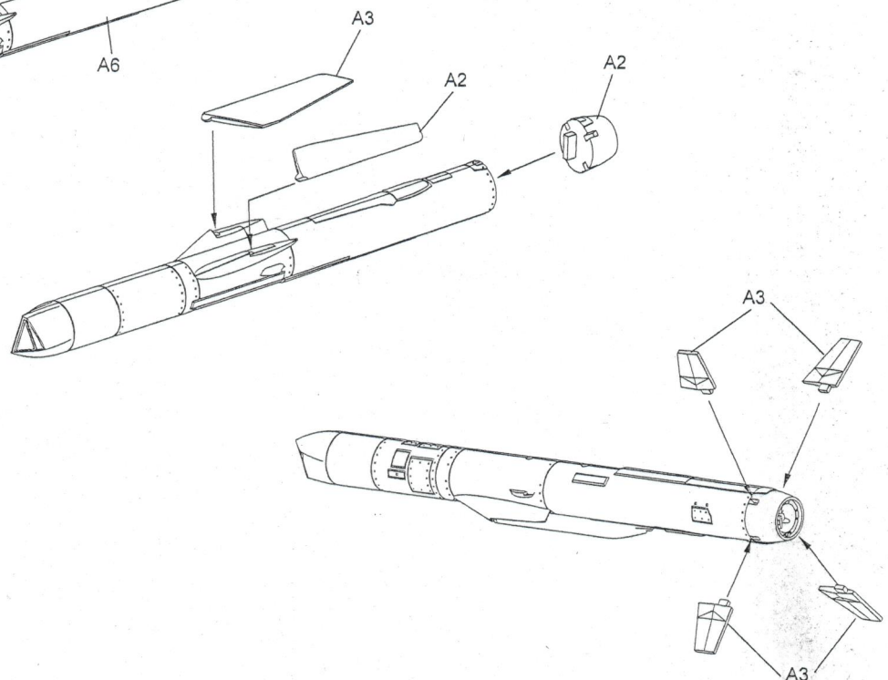
AGM - 84H SLAM - ER
