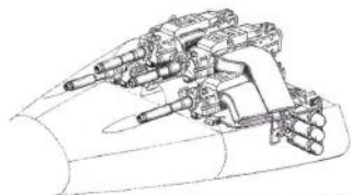
◆MK108 30mm機関砲
