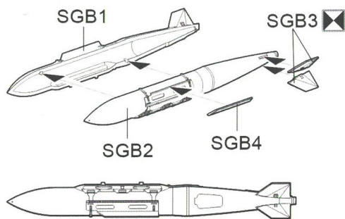
GBU-31-V3
