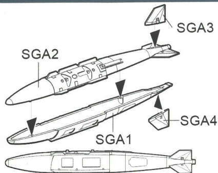
GBU-31-V1
