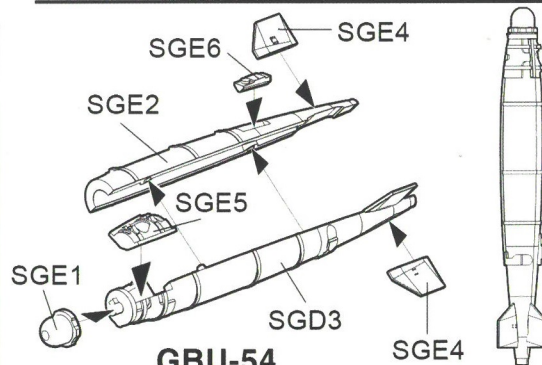
GBU-54
