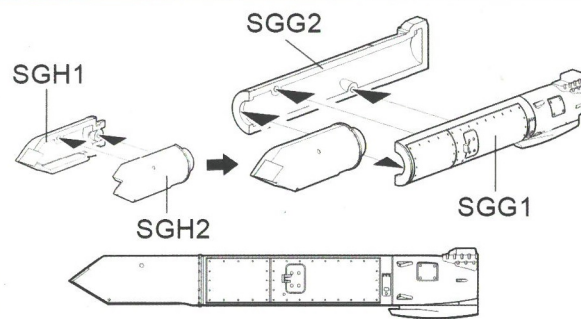
ANAAQ-33
