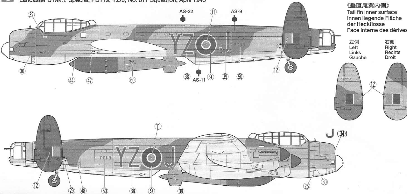
C PD119 YZ/J 第617飛行隊所属 ランカスター B Mk.Iスペシャル 1945年4月 Lancaster B Mk.I Special, PD119, YZ/J, No. 617 Squadron, April 1945
