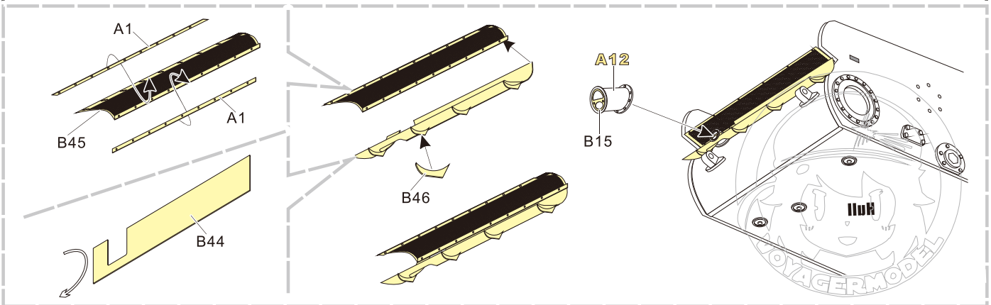
KV-2 Mod 1939 KV-2 1939型
