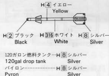
武装搭載図
