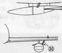
増槽支柱取り付け参考図
