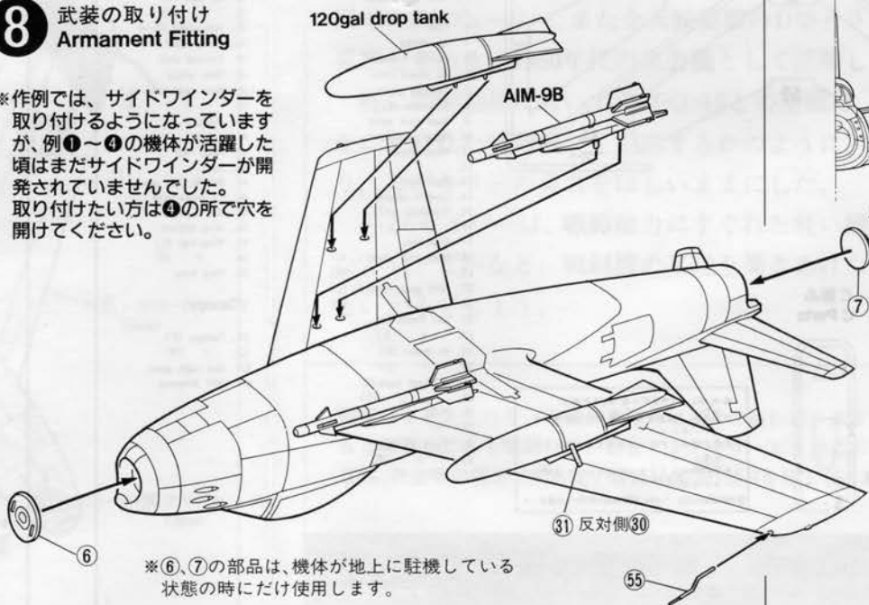
武装搭載図
