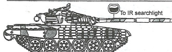
T-72B of Russian Army, central Russia, 2002. T-72Б ВС России, 2002.
