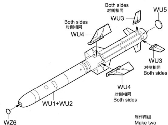
《AGM-84E》
