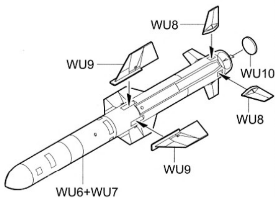
《AGM-84A》
