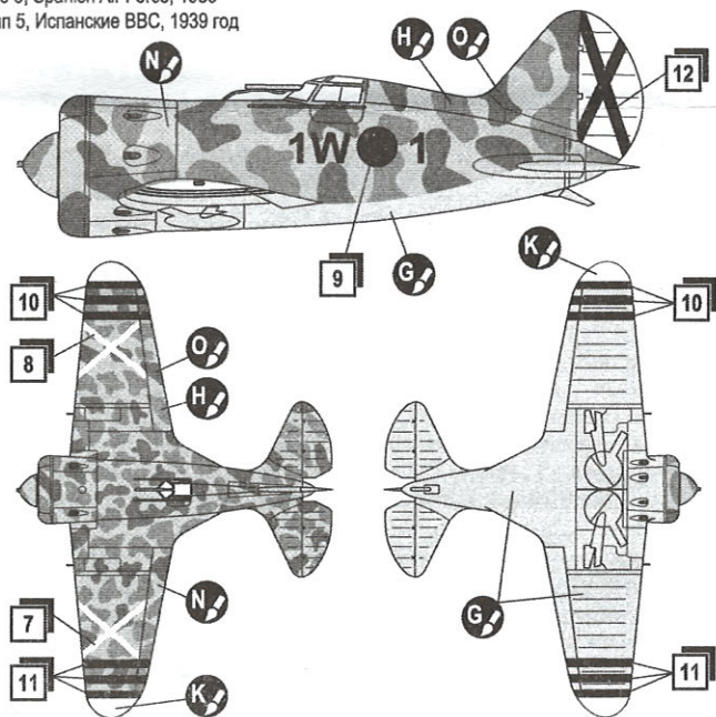
I-16 type 5, Spanish Air Force, 1939 И-16 тип 5, Испанские ВВС, 1939 год
