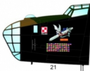
Liberator GR V, BZ965 pod koniec służby w 1586 S.E. Do Z.S., marzec 1945 roku Liberator GR V, BZ965 at final stage of service in 1586th SDF
