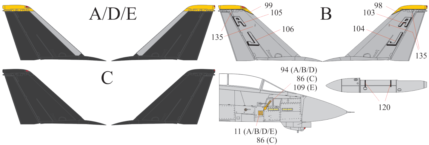
E. F-14A-95GR Tomcat, 1980.
