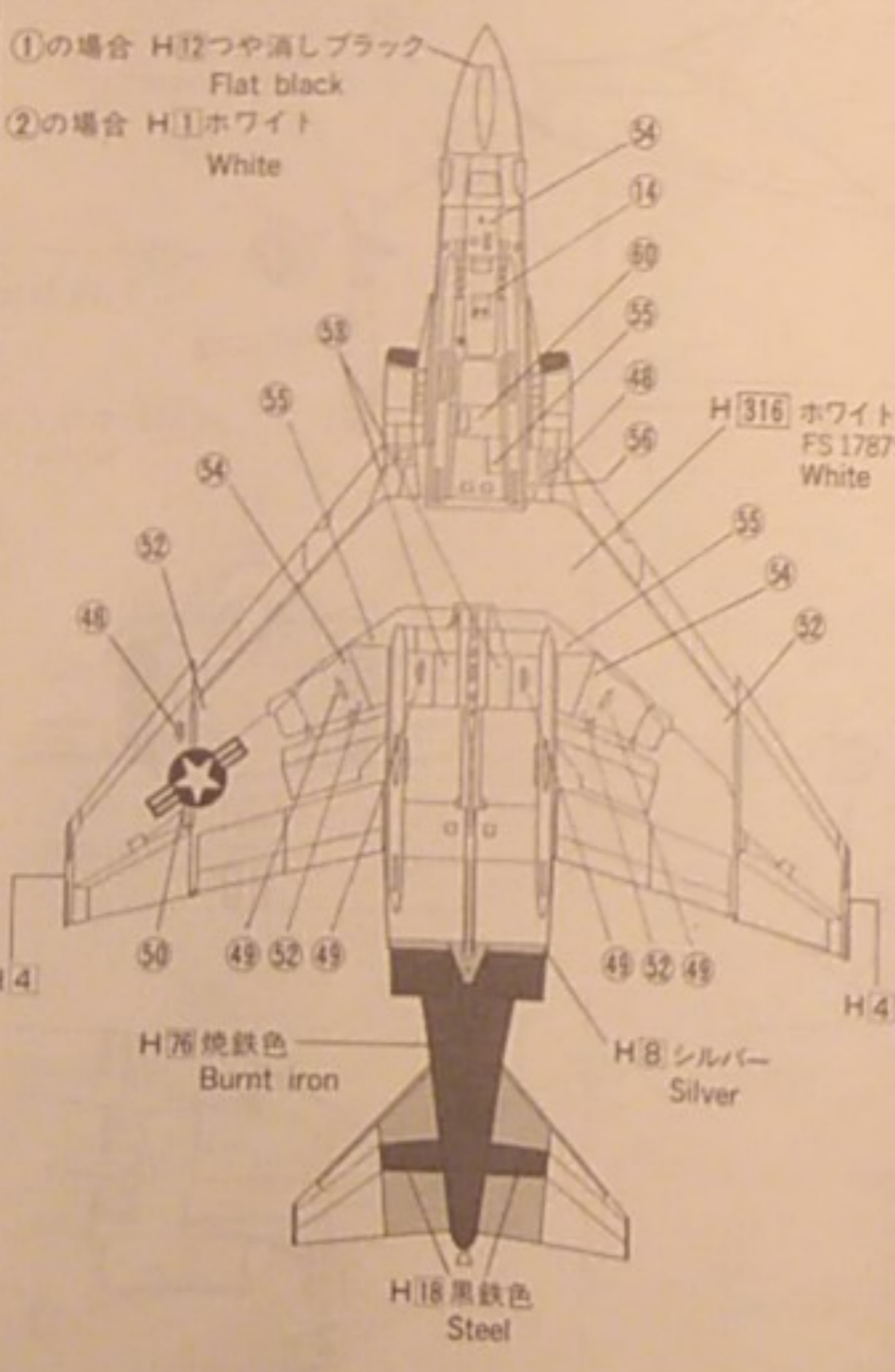
〈下面 BOTTOM VIEW〉
