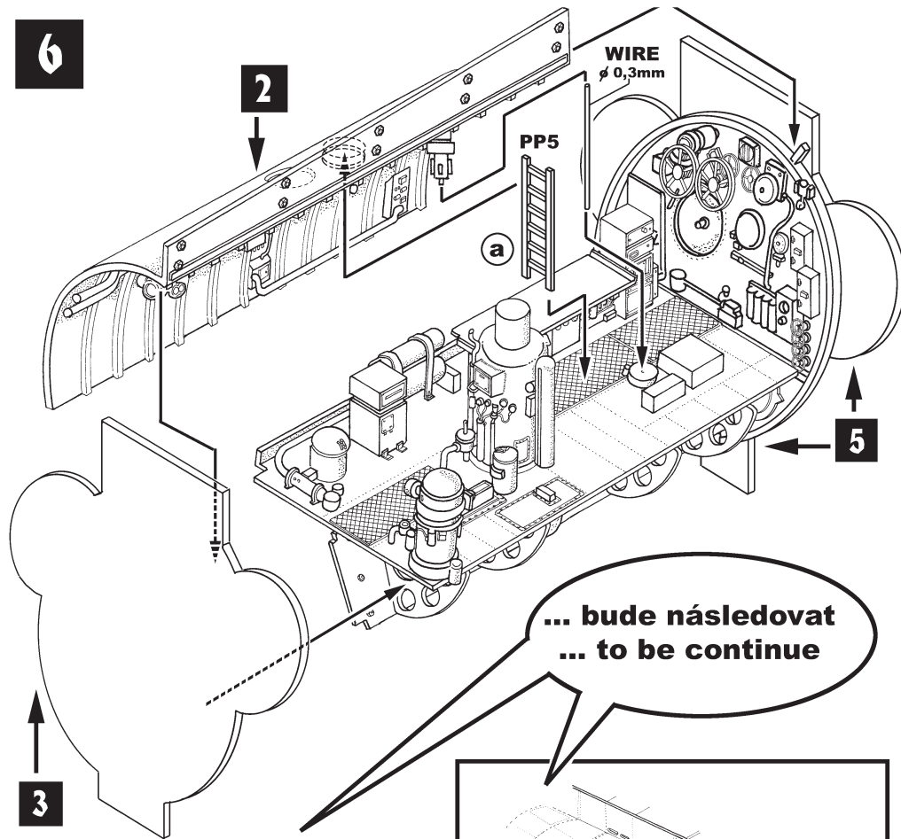
N72002 Torpédová sekce Torpedo section
