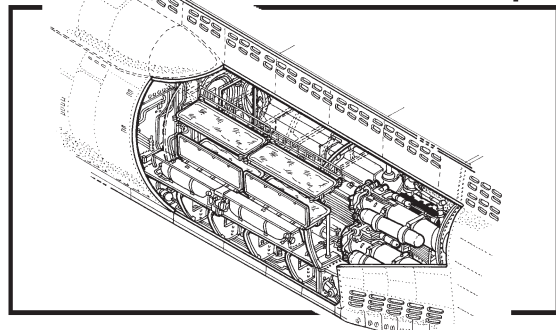
N72002 Torpédová sekce Torpedo section
