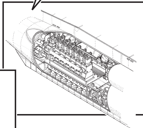
N72003 Motorová sekce Engine section
