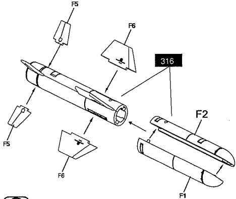
AGM - 84D HARPOON
