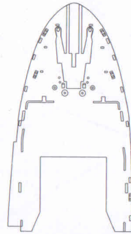
前机库甲板 Fore hangar deck
