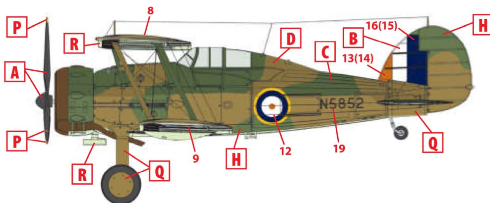
3. Gloster Gladiator Mk.II, 1-я эскадрилья SAAF, Восточная Африка, 1940 г. Gloster Gladiator Mk.II, No 1 Squadron SAAF, East Africa, 1940
