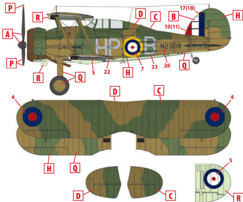
1. Gloster Gladiator Mk.II, 247-я эскадрилья RAF, Роборо, август 1940 г. Gloster Gladiator Mk.II, No 247 Squadron RAF, Roborough, August 1940
