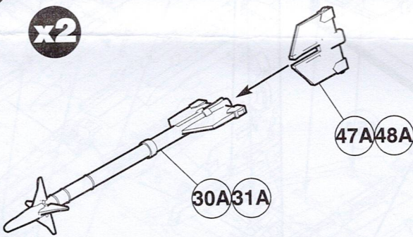
AIM-9L SIDEWINDER
