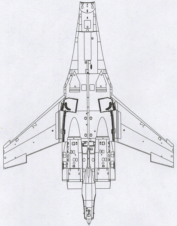
《下部机身》 Lower fuselage
