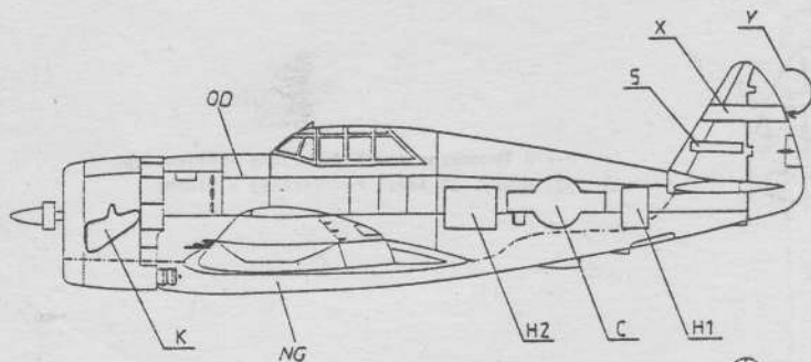
P-47 D-20RF Thunderbolt z 361 dywizjonu myśliwskiego 356 Grupy 8 Armii Powietrznej. A Pilot Lt. Thomas Bailey
