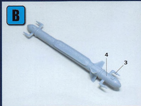
(B) AN/ALQ-167(V)70/72
