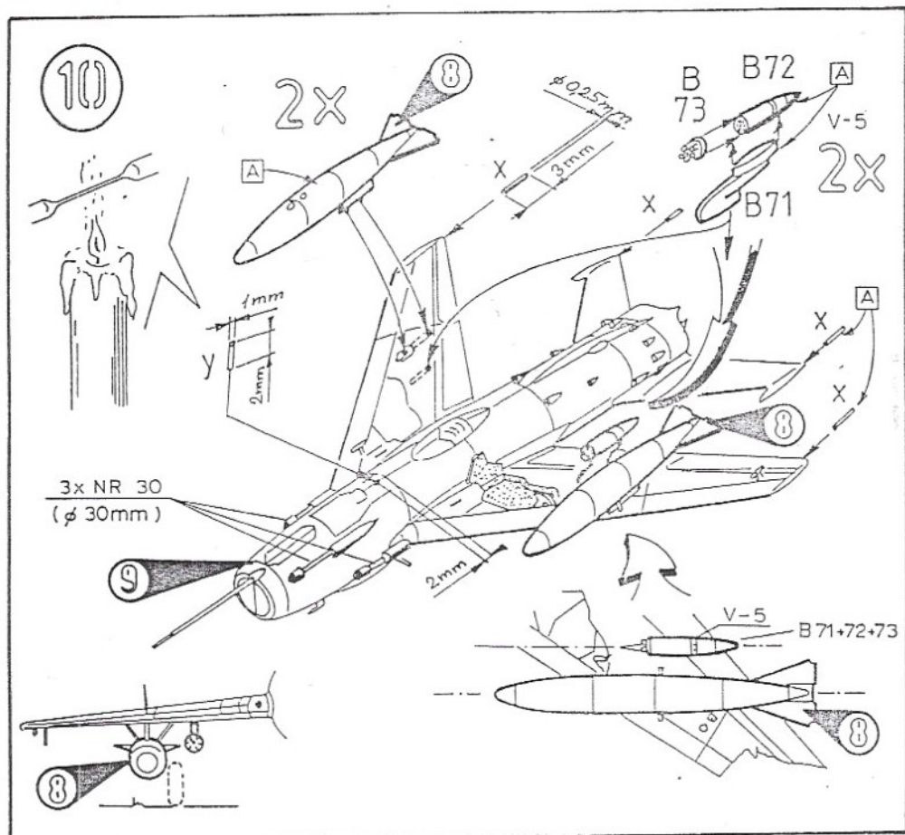
ROCKET POD V-5 RAKETNICE V-5 (8x ø 57mm)
