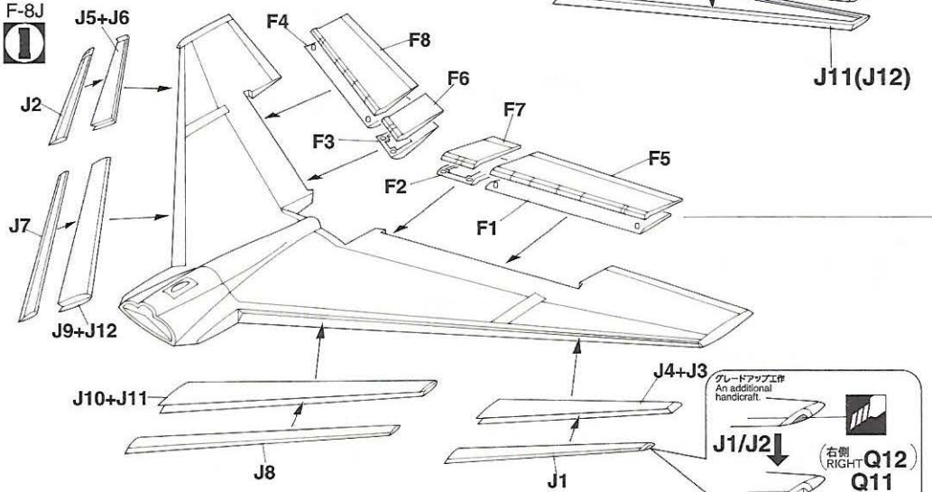
主翼を下げた状態 Main Wing Down
