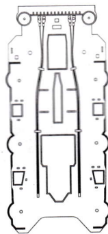
《中甲板》 Center deck
