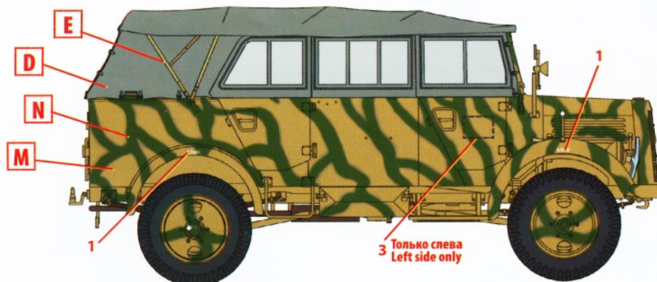
4. L1500A, Италия, лето 1944 г. L1500A, Italy, Summer 1944
