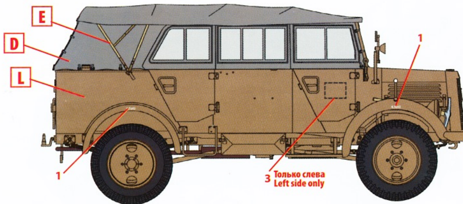
3. L1500A, Северная Африка, лето 1942 г. L1500A, North Africa, Summer 1942
