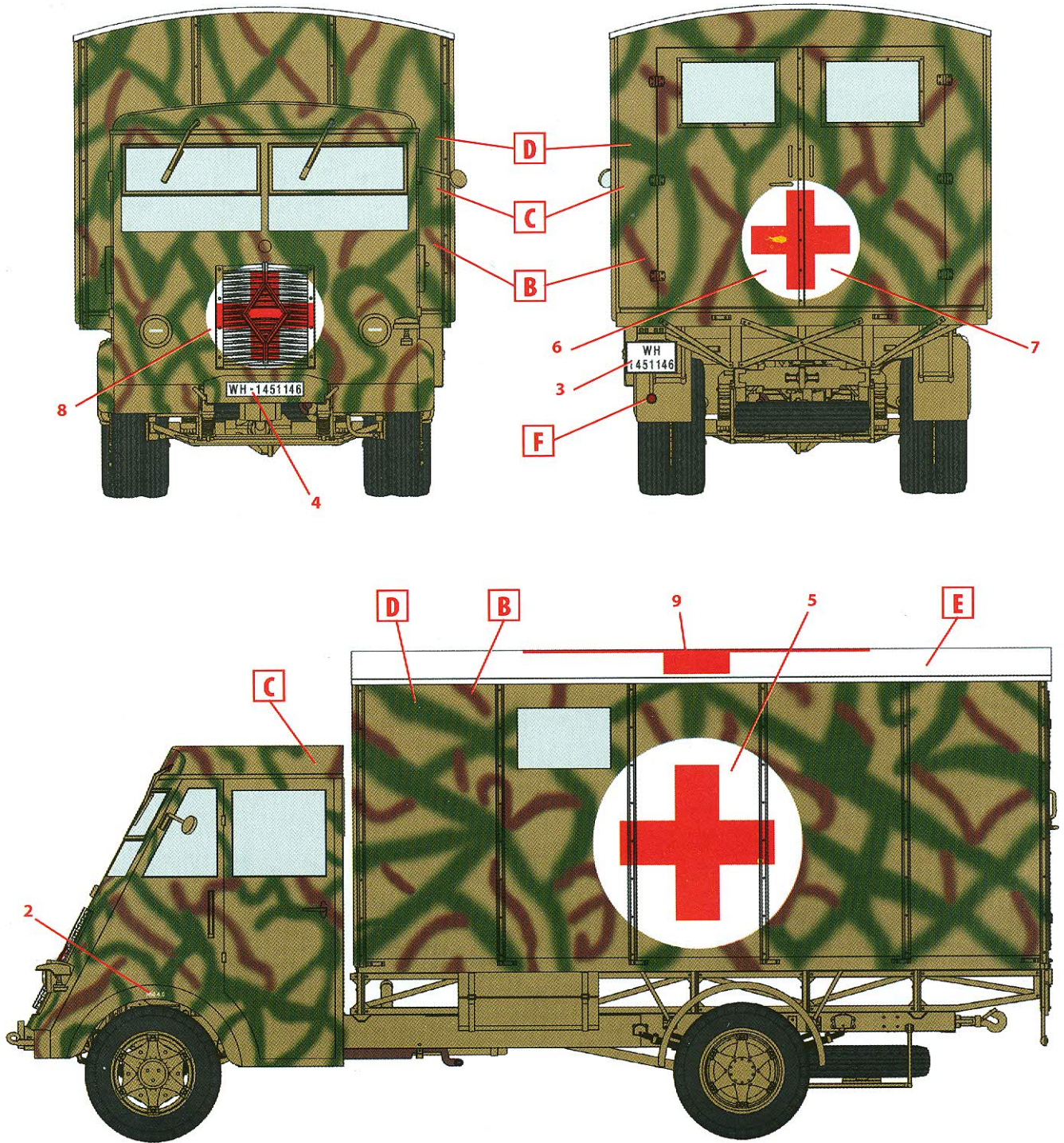
Lastkraftwagen 3,5 t AHN с закрытым кузовом, Франция, 1944 г. Lastkraftwagen 3,5 t AHN with Shelter, France, 1944
