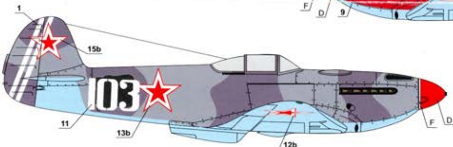
14. Як-3 предположительно командира 402 иап 265 иад полковника А.Е.Рубахина, 1-й Белорусский фронт, 1945г. 14. Yak-3 probably of Col A.E.Rubakhin, CO of 402 fighter regt, 265 fighter division, First Belorussian Front, 1945
