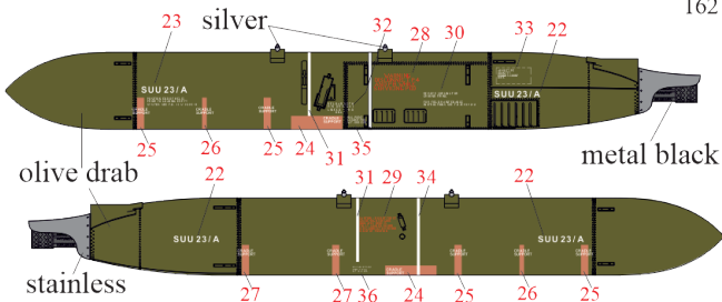
SUU-23/A for RAF(FGR.2)
