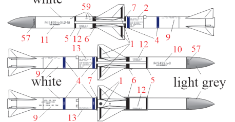
AIM-7E for RN & RAF (FG.1)
