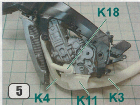
5 写真の通りパーツを組みます。
