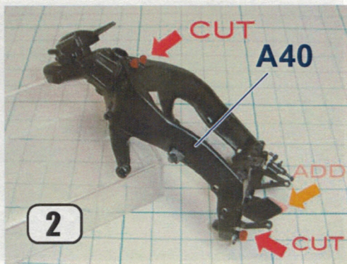
2 左ステップホルダーの板をプラ板等で形状変更します。
