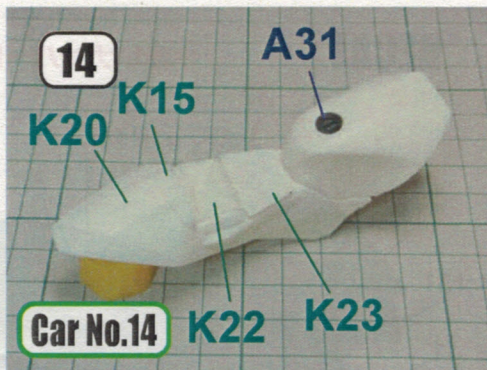
ゼッケン#13号車の場合。 K23をカットして使用します。
