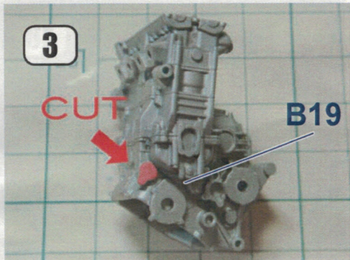
3 写真の部分をカットします。
