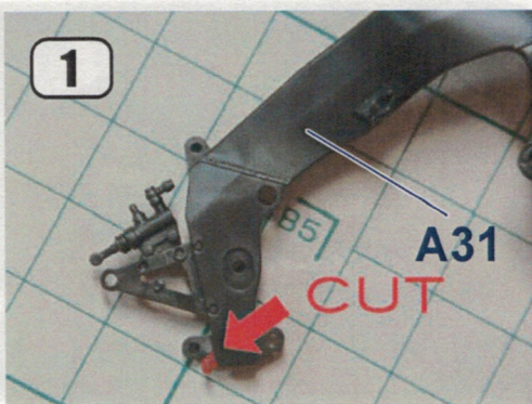
1 写真の突起物をカットします。
