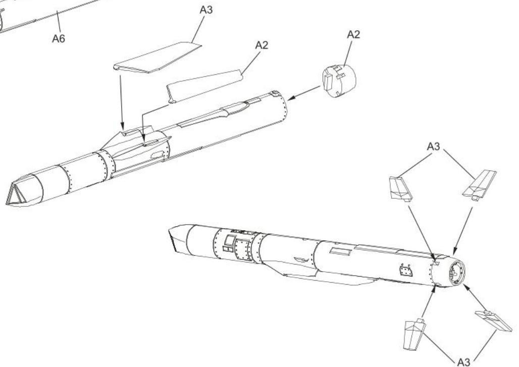
AGM - 84H SLAM - ER
