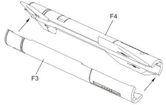
AGM - 84D HARPOON
