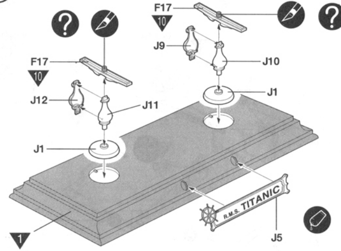
STAND HALTERLING SUPPORT 座台 받침대
