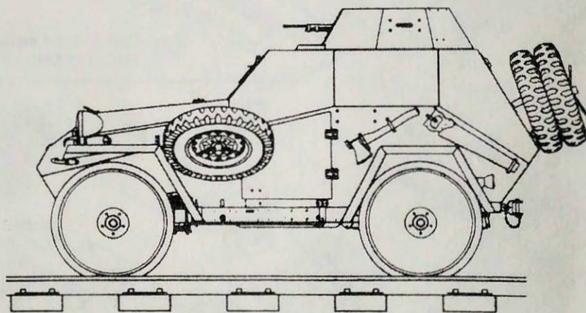
BA-64V (Vyksunsk) Red Army, 1943. Russian khaki-green (4BO). БА-64В (Выксинский) Красная Армия. 1943. Хаки (4Б0).
