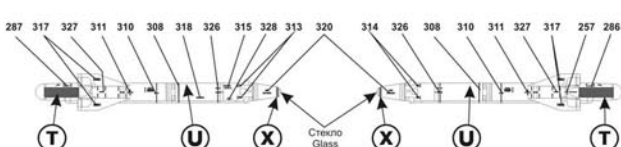
Управляемая ракета "Воздух-Поверхность" типа X-25МП x 4 Kh-25ML Air to Surface missile x 4
