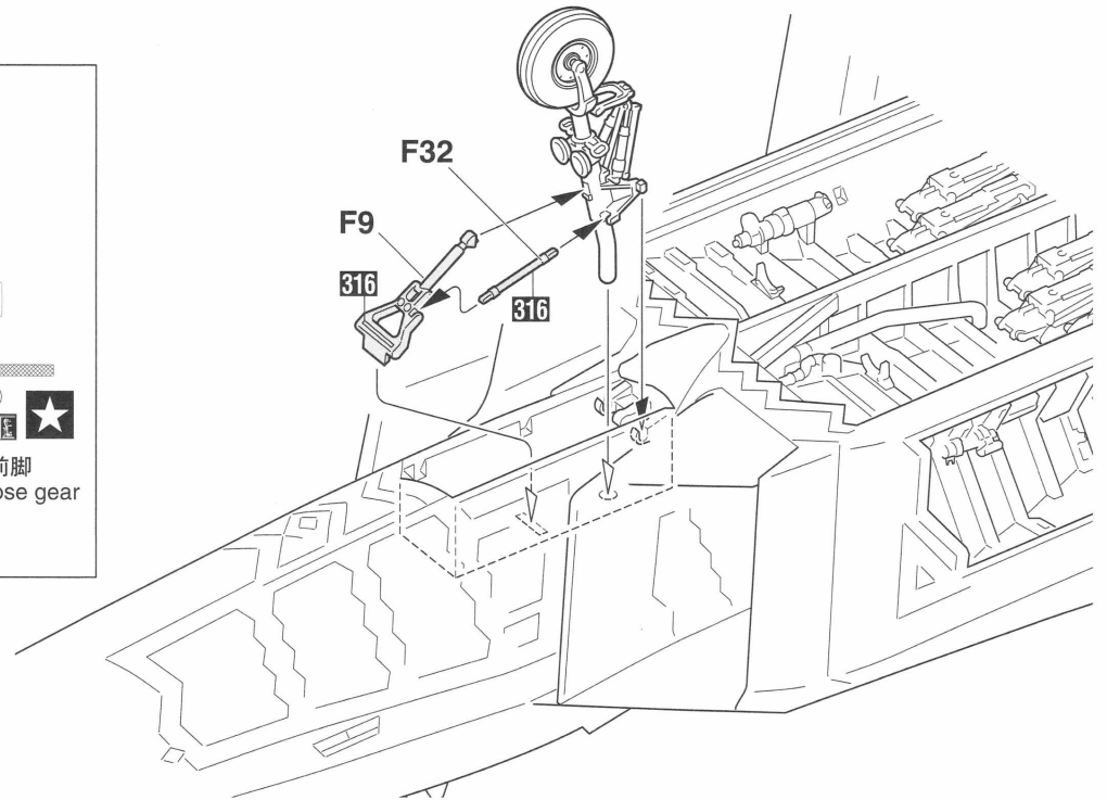
前脚取り付け参考図 Nose gear installation reference chart
