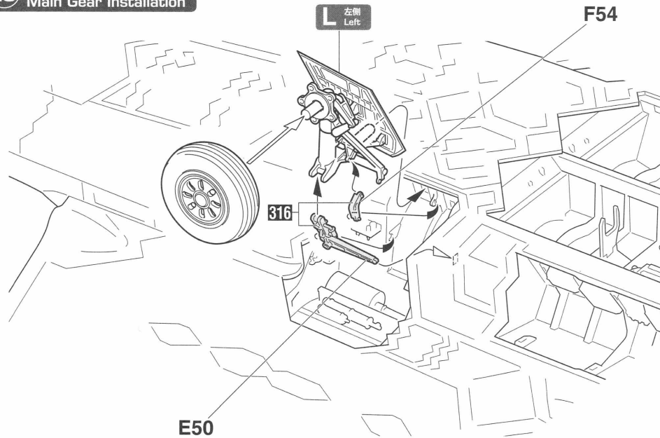
左主脚取り付け参考図 Left Main gear installation reference chart
