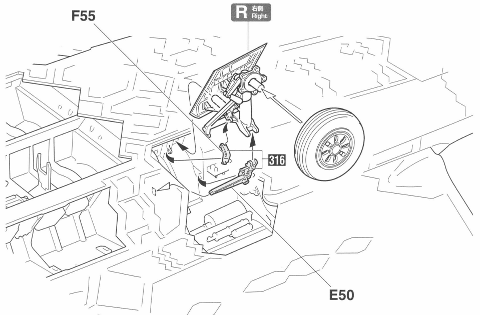
右主脚取り付け参考図 Right Main gear installation reference chart
