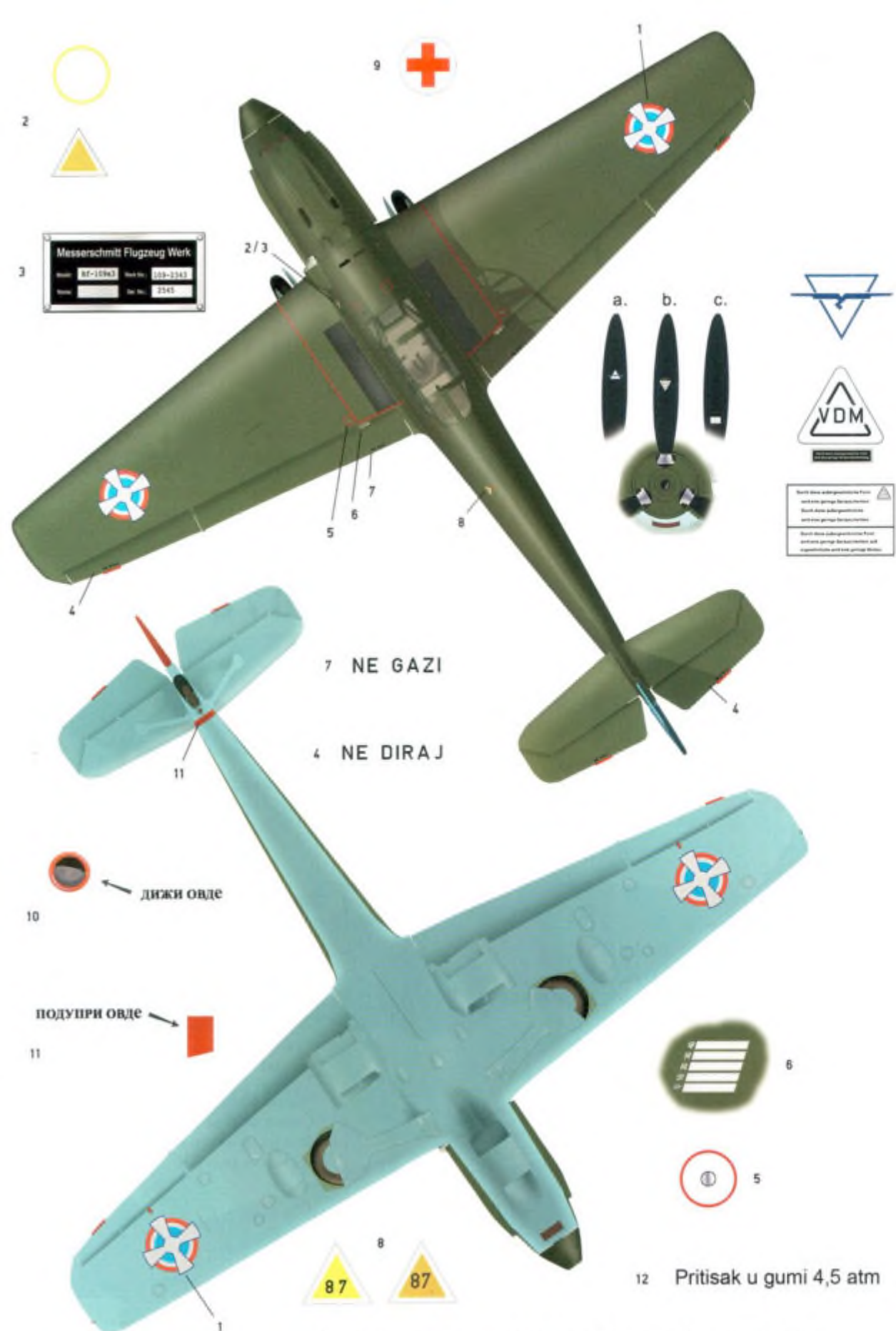
Vues de dessus et de dessous des Me-109 E-3a yougoslaves, avec les divers marquages et leurs emplacements sur l'appareil.
