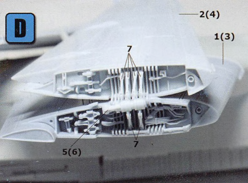
(D) Actuators
