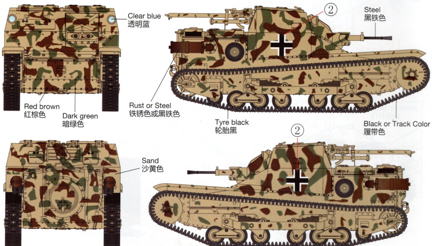
Option 2: German captured vehicle, unit unknown, Italy 1943. 1943年间在意大利境内德军缴获之车辆。
