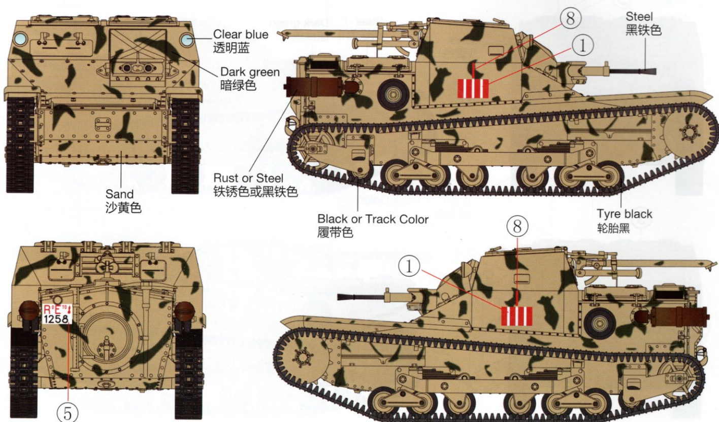
Option 3: The Special Armoured Brigade of the XXIIIrd Corps, 5th Army, Libya, 1940. 1940年在北非利比亚作战之意大利第五军团第23兵团之特别装甲旅属下车辆。
