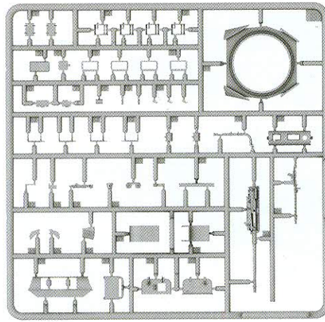
Frame J / Ramka J
