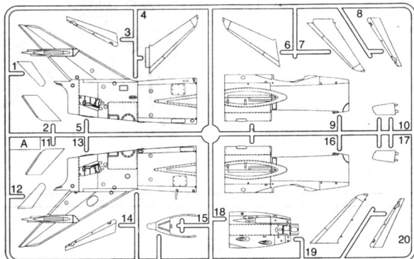
部品图 (Parts)
