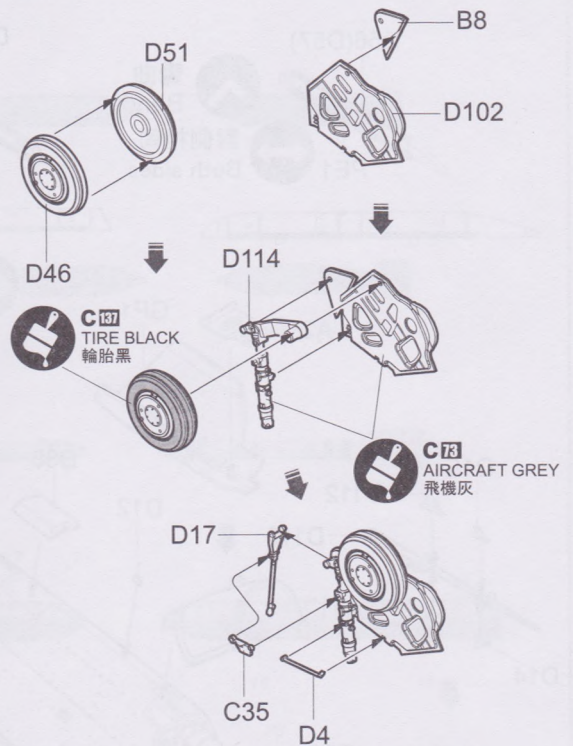
《左側起落架》 Left undercarriage
