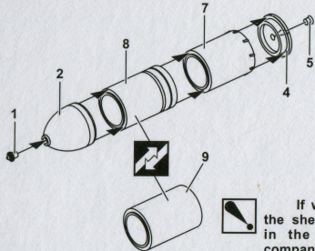
Raketen Sprenggranate 4581
