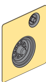
使用遮喷板为轮毂 喷上所需要的颜色 use template to paint required hub colour
