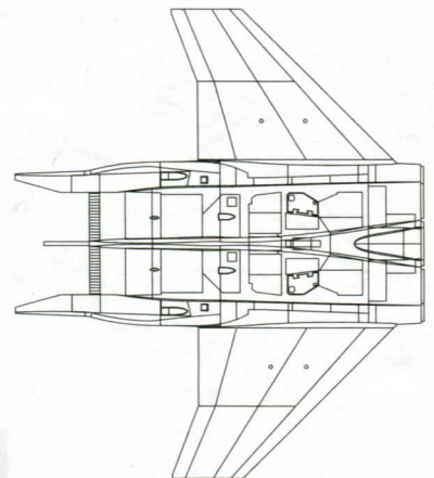
<<下部机身>> Lower Fuselage
