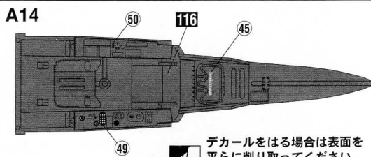
計器板、コックピット後部 Instrument panel and the back of cockpit
