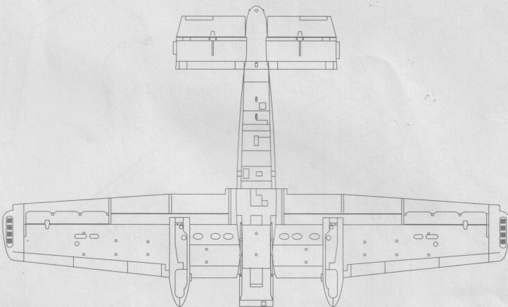
<<下机翼>> Lower wing
