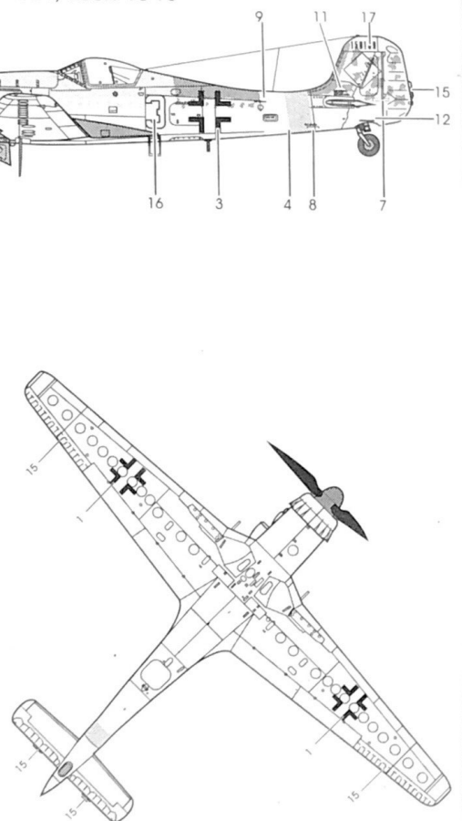
Ta 152 H, JG 301, Leck 1945
