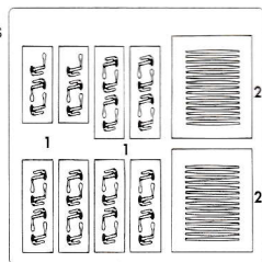
《MA》 エッチング部品 PHOTO-ETCHED PARTS
