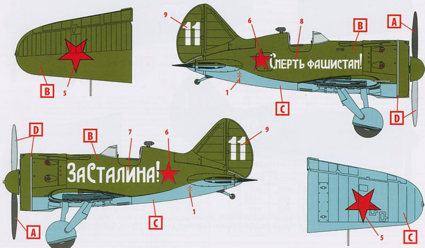
2. И-16 тип 24, 72-й САП ВВС Северного флота, лето 1941 г. I-16 type 24, 72d Mixed Regiment of the Northern Fleet Aviation, Summer 1941
