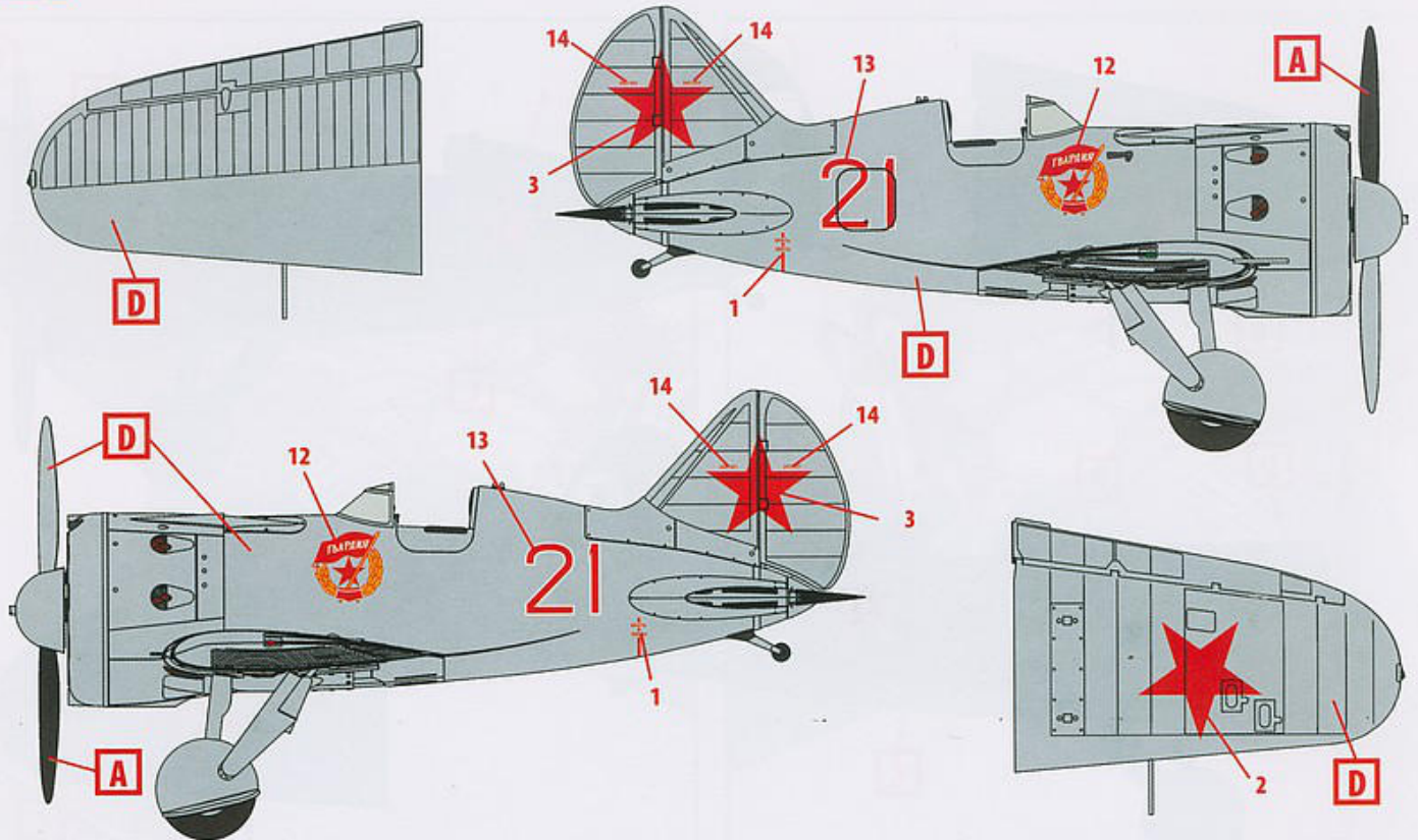
3. И-16 тип 24, 4-й ГвИАП ВВС Балтийского флота, зима - весна 1942 г. I-16 type 24, 4th Guard Fighter Regiment of the Baltic Fleet Aviation, Winter - Spring 1942
